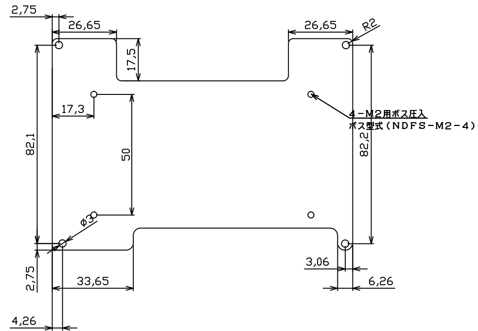
液晶押え板 AL t1.0
