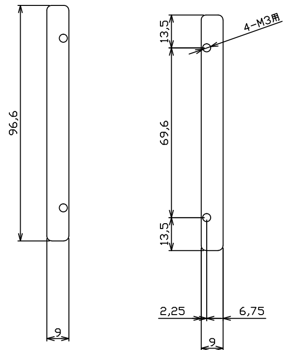
取付板 sus t1.5
