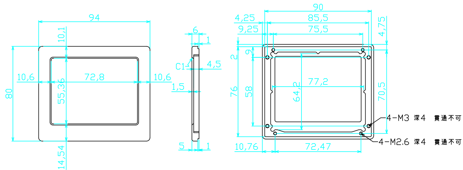
フレーム A5052 t6.0
