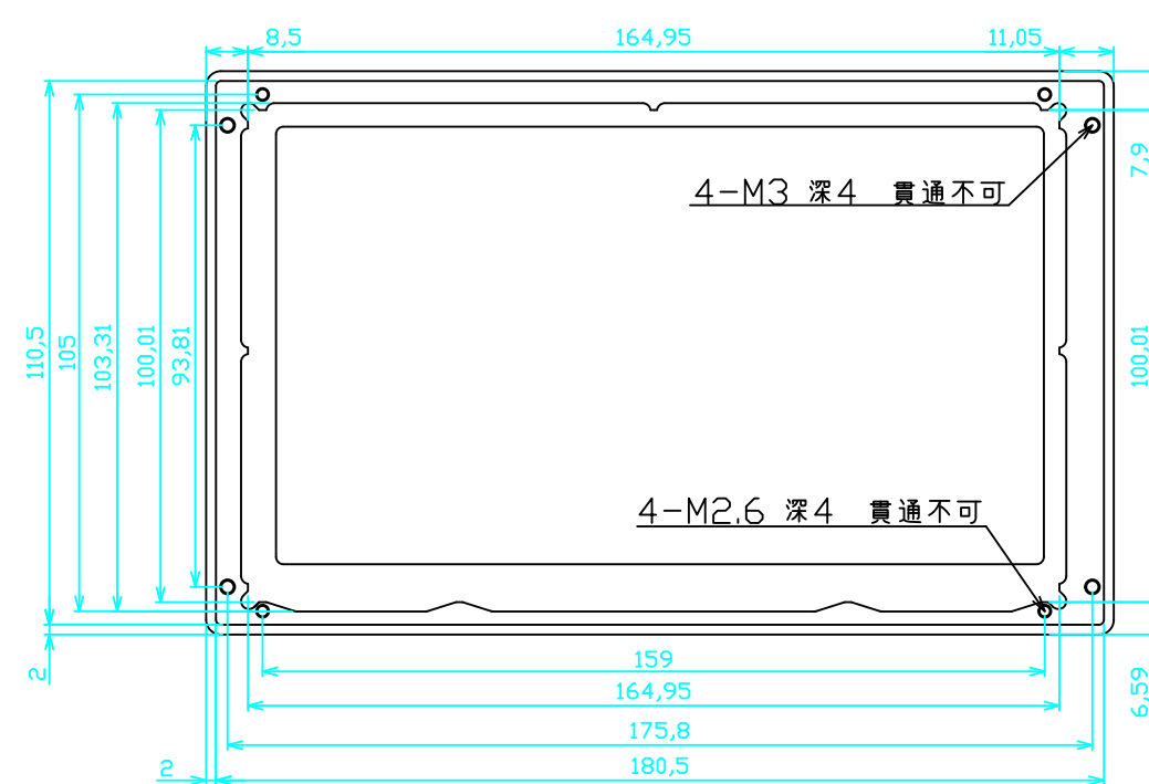
フレーム A5052 t6.0
